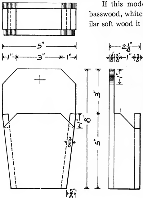
Fig. 272—Whisk Broom Holder
